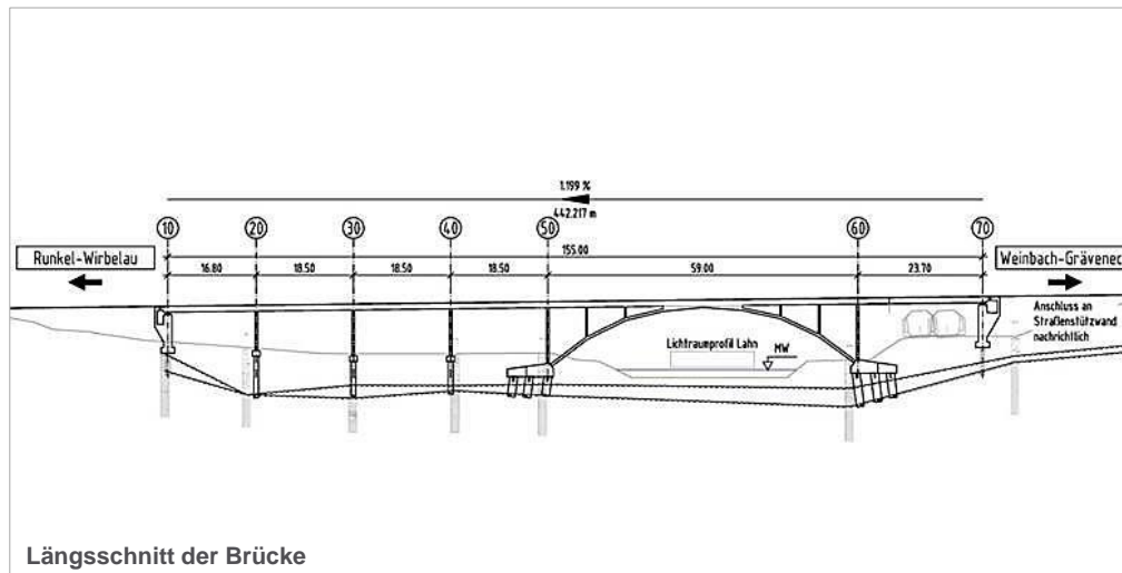
Bestandsbrücke
