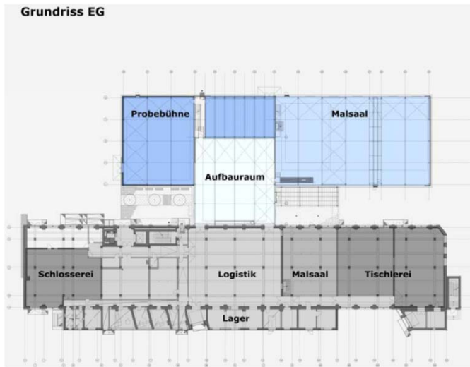
Grundriss EG
