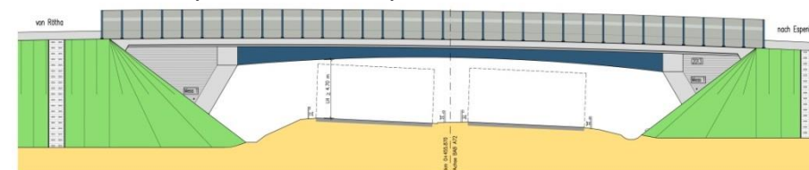
Ansicht BW 61Ü1 (Stützweite 42 m / 38 m)
