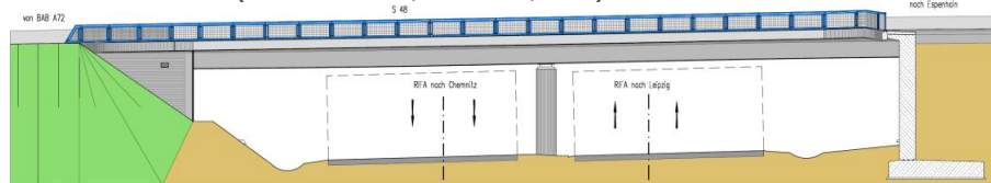
Ansicht BW 59.1 (Stützweite 25,20)
