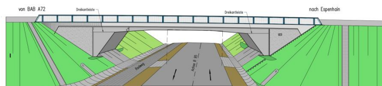
Ansicht Brücke 59.2 (Stützweite 10,45 m)
